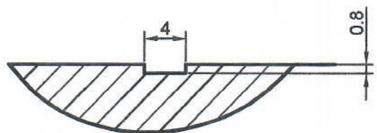
Presjek "A - A" M 2:1
