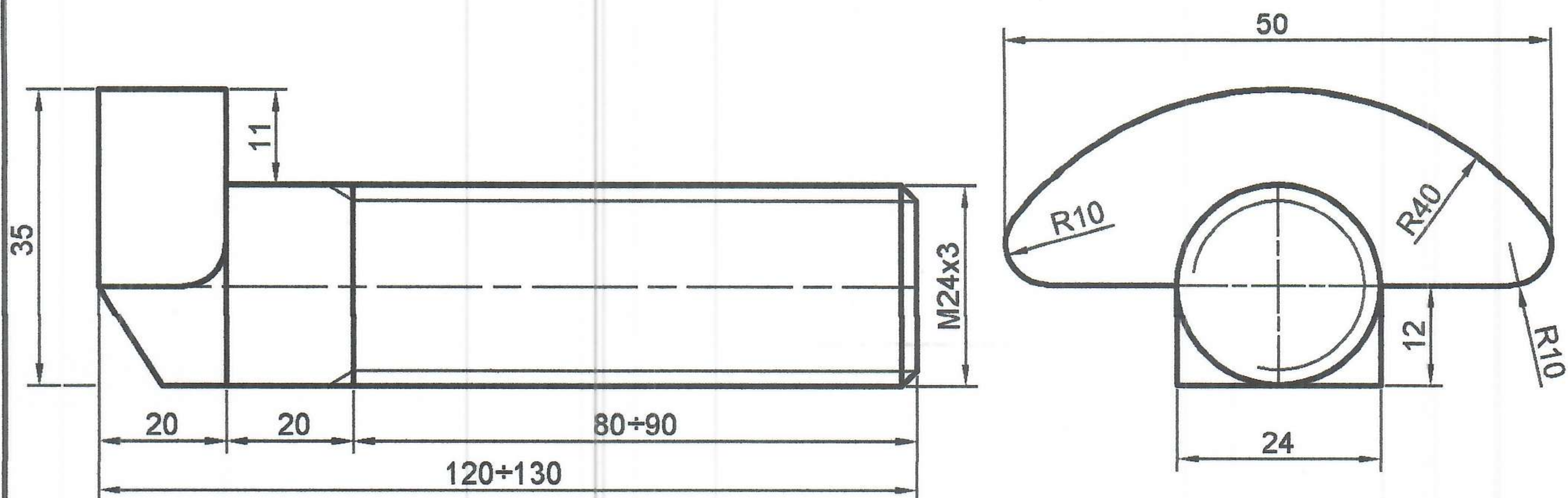
Vijak TH-29 (M24x3x90) Kvalitet vijka 8.8
